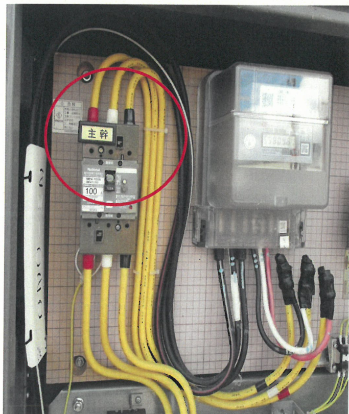
③ 主幹ブレーカー
