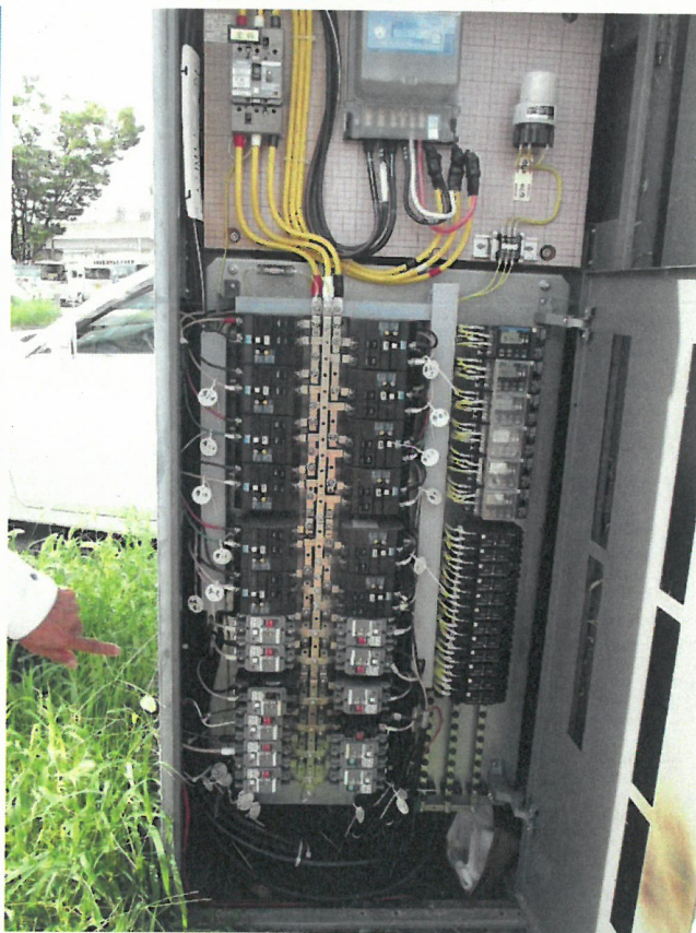
② 分電盤 内部
