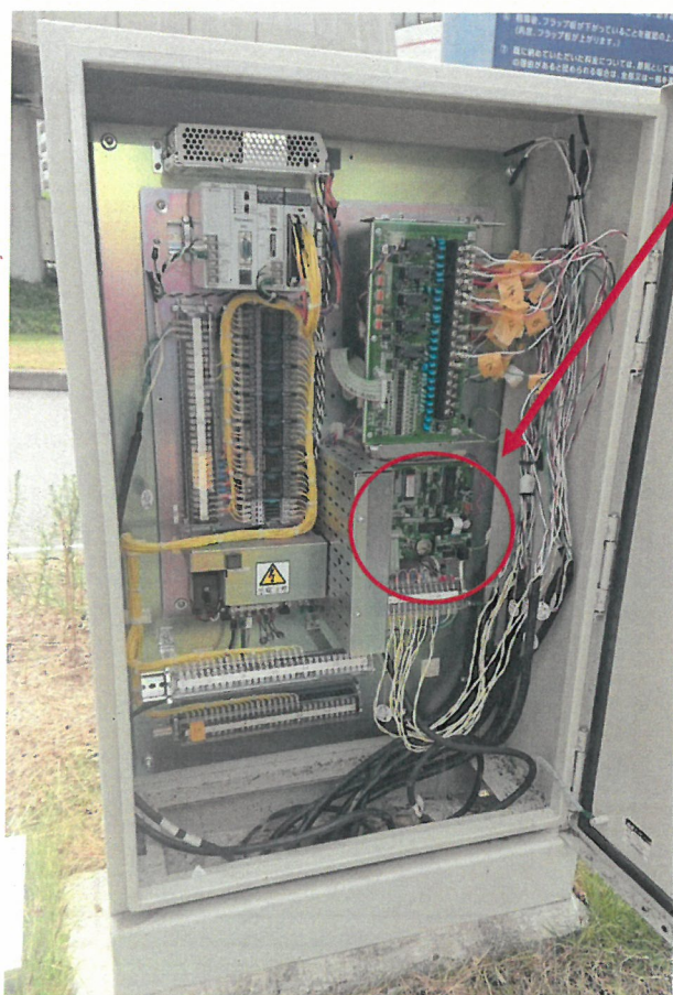
⑦ 分電盤内部
