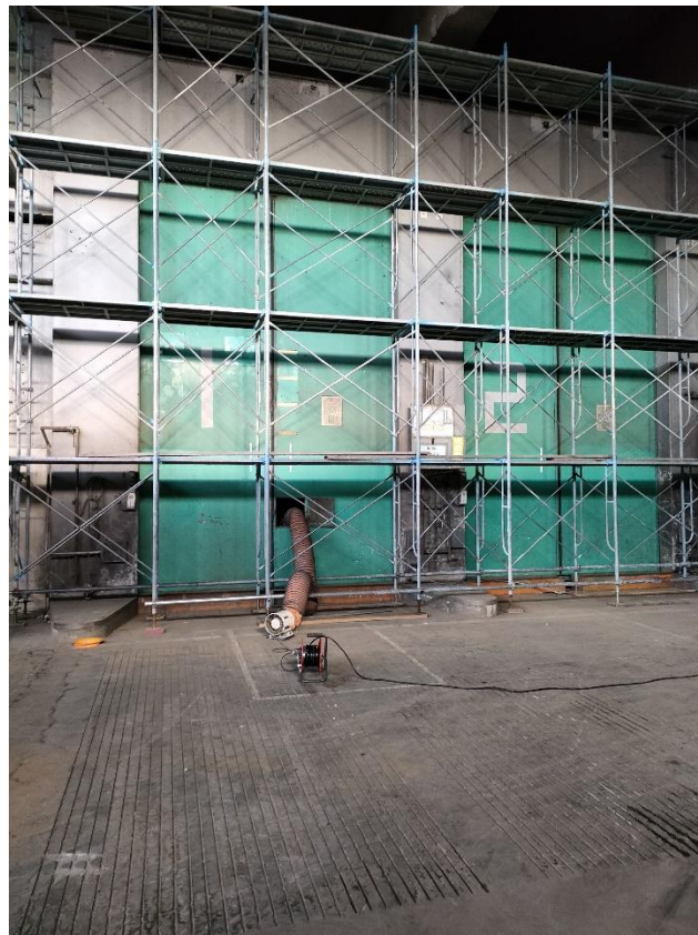
【プラットフォーム足場設置状況】
