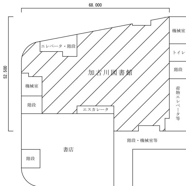
6階配置図 縮尺 1/1,000 単位(m)
