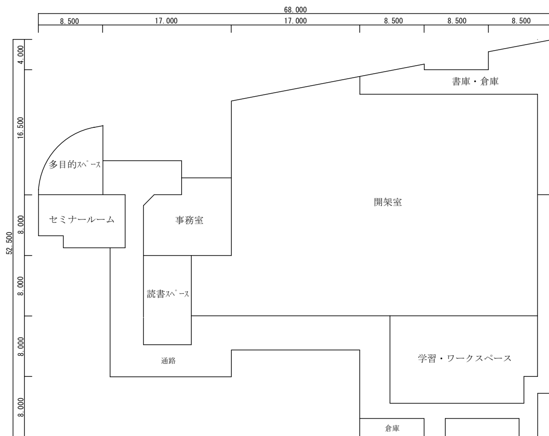
平面図 縮尺 1/500 単位 (m)
