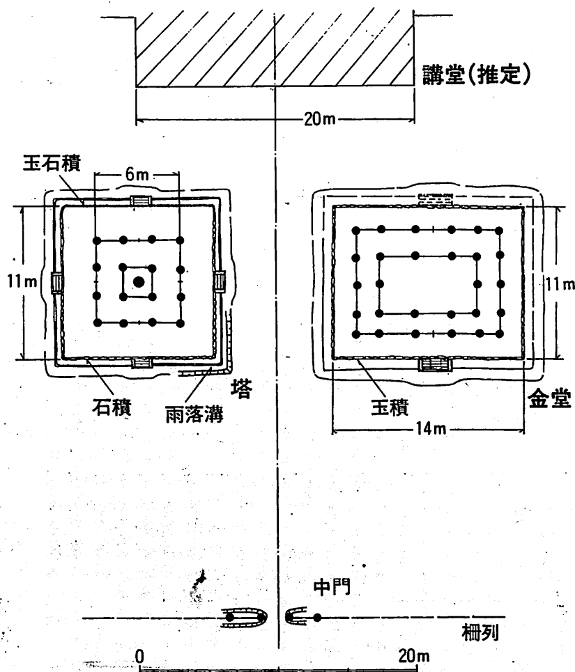
伽藍配置平面図
