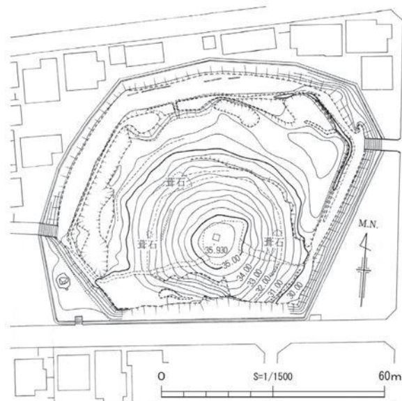
北大塚古墳墳丘測量図 (高野 1996 をもとに作成)
