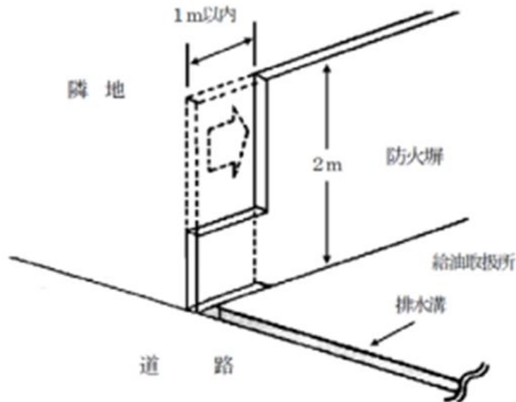
【切欠きの例】
