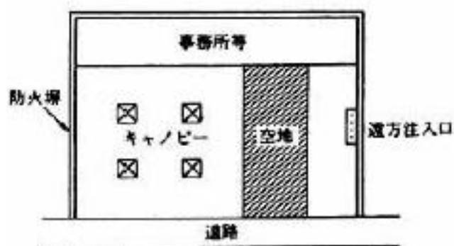
【避難空地を給油取扱所の端にとらない場合】
