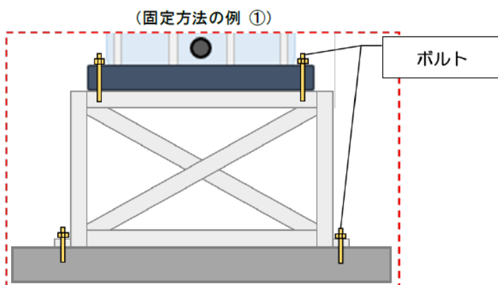
【重力により払い出すタイプの設置例】
