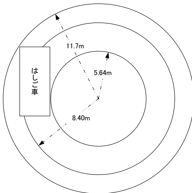
図6 (はしご車の最小回転に必要な空地の算出)
