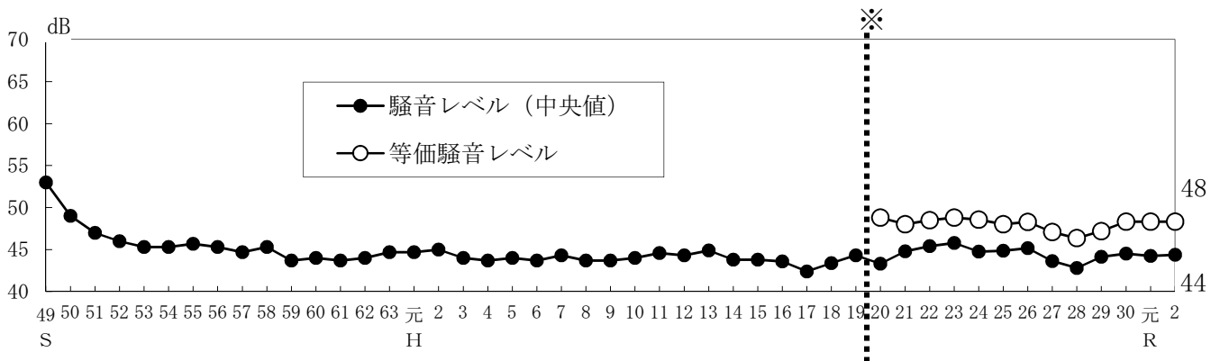
図-10 住居地域（東、中、西門）における騒音の経年変化（23時～翌朝5時）
