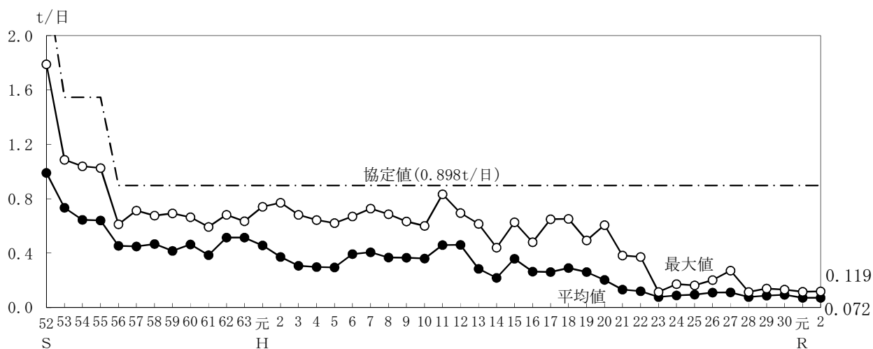
図-7 SS負荷量の推移
