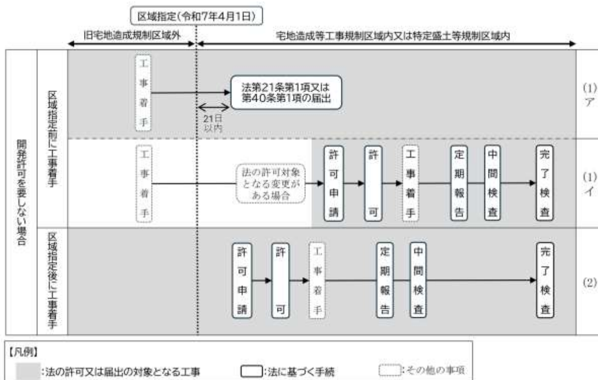
図3-16-1 旧宅地造成規制区域外であって開発許可が不要な場合の手続のイメージ
