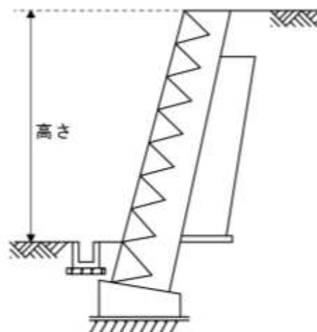
図 1－1－5 擁壁の高さ
