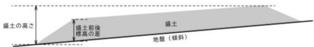
図1-1-2 盛土の高さ及び盛土前後の標高の差のイメージ図
