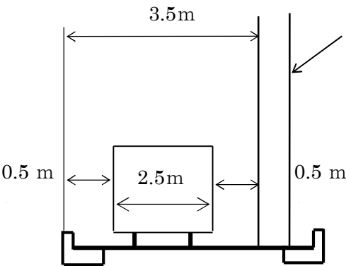
局所的道路占有物 (電柱等)
