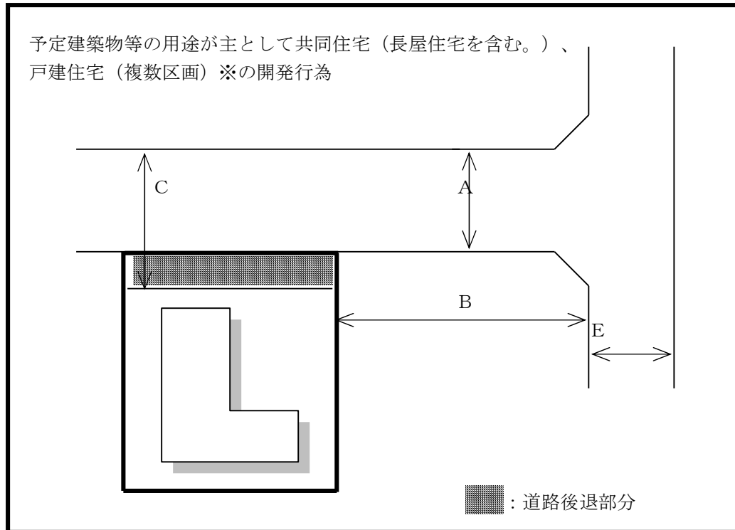
ウー 1 予定建築物等の用途が住宅の場合の例 (図 7-1)
