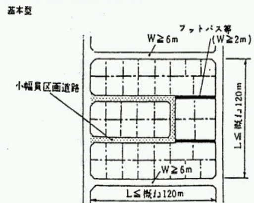
4) U 字状小規模区画道路
