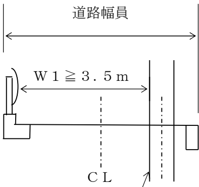
局所的道路占有物 (電柱等)
