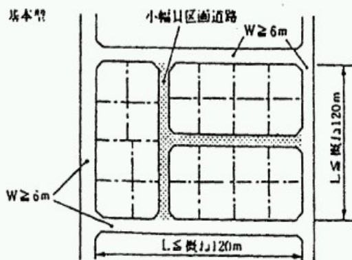
3) T 字状小規模区画道路
