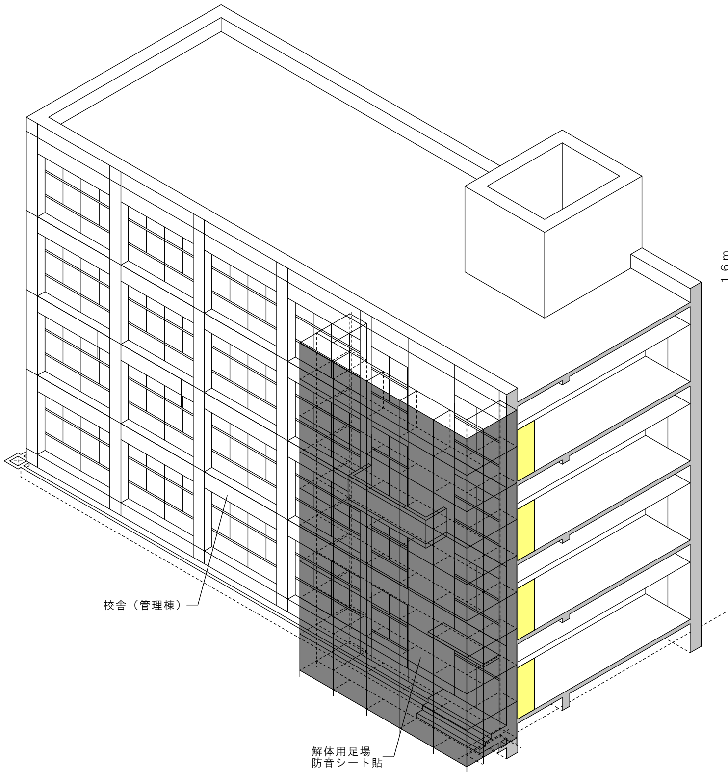
バルコニー・庇・建具撤去工事の際の校舎の状況
