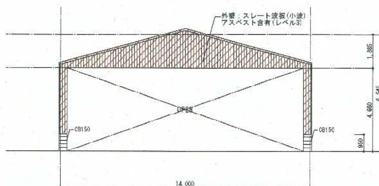
西立面図 1:100
