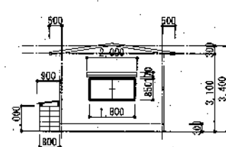
西立面図 1:100
