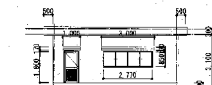
南立面図 1:100
