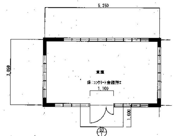
平面図 1:50
