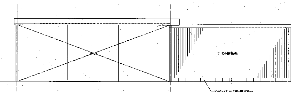
B棟 南立面図 1:50
