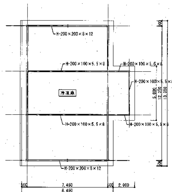
天井伏図 1:100
