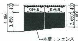
東立面図 1:200
