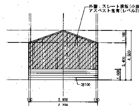
南立面図 1:100
