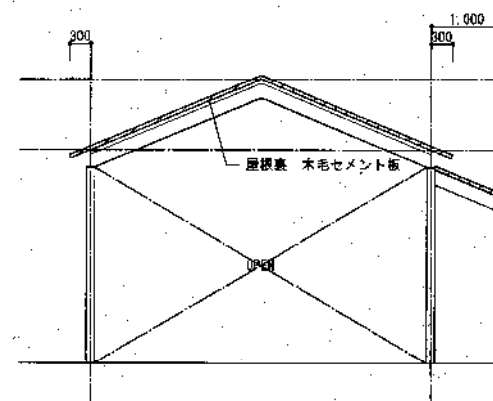
A棟 西立面図 1:50
