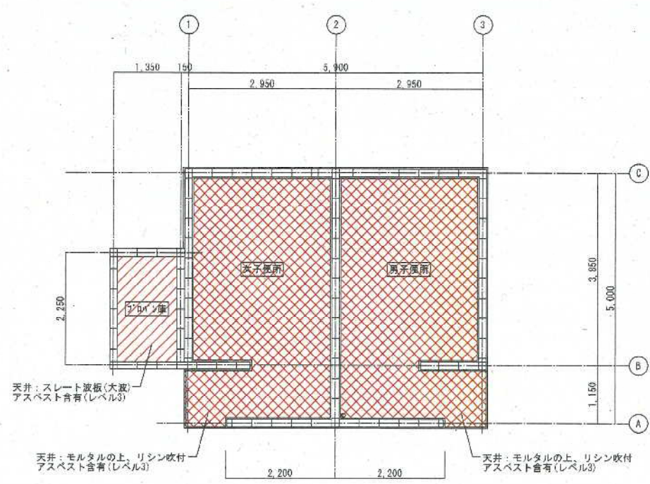
天井伏図 1:50
