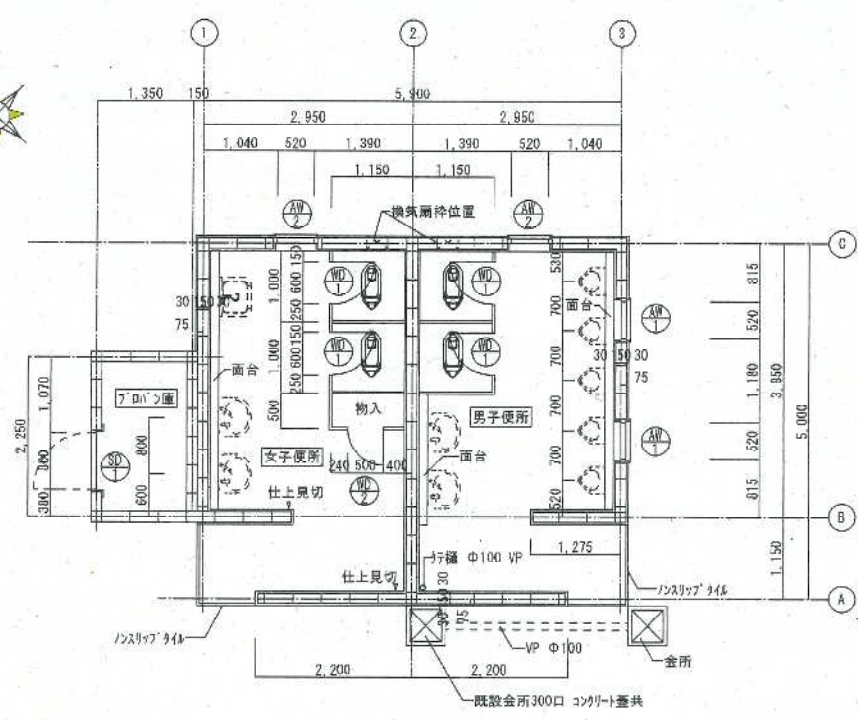
平面図 1:50
