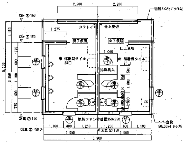
平面図 1:50
