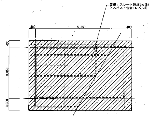
屋根伏図 1:50
