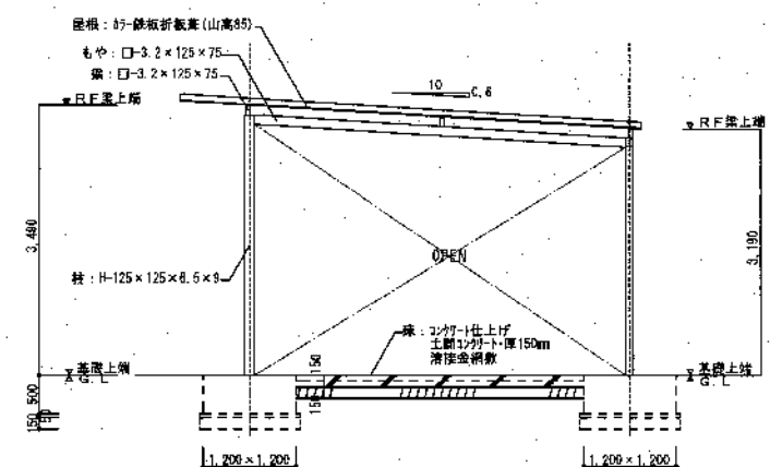
断面図 1:50
