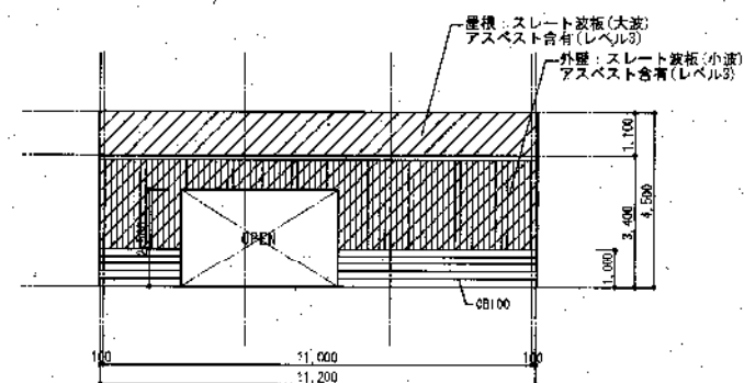
東立面図 1:100
