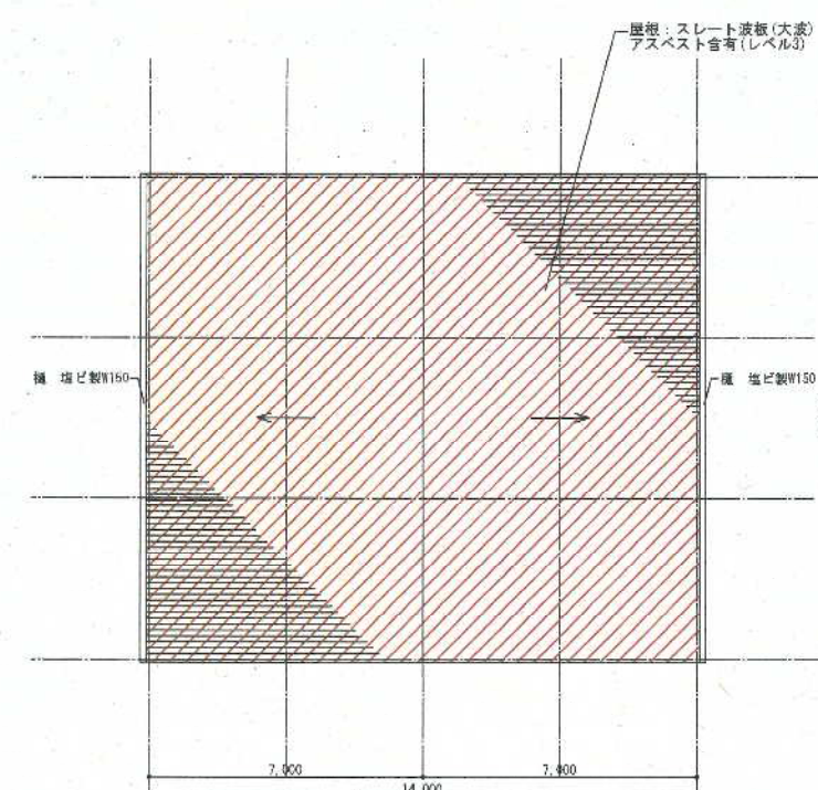
屋根伏図 1:100
