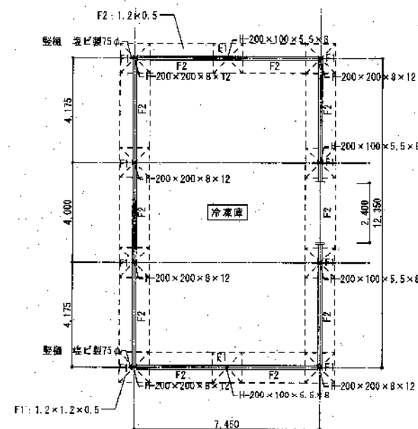
1階平面図 1:100
