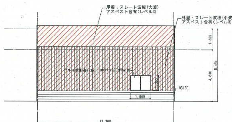
南立面図 1:100
