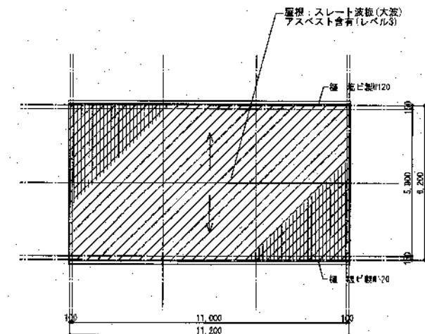
屋根伏図 1:100
