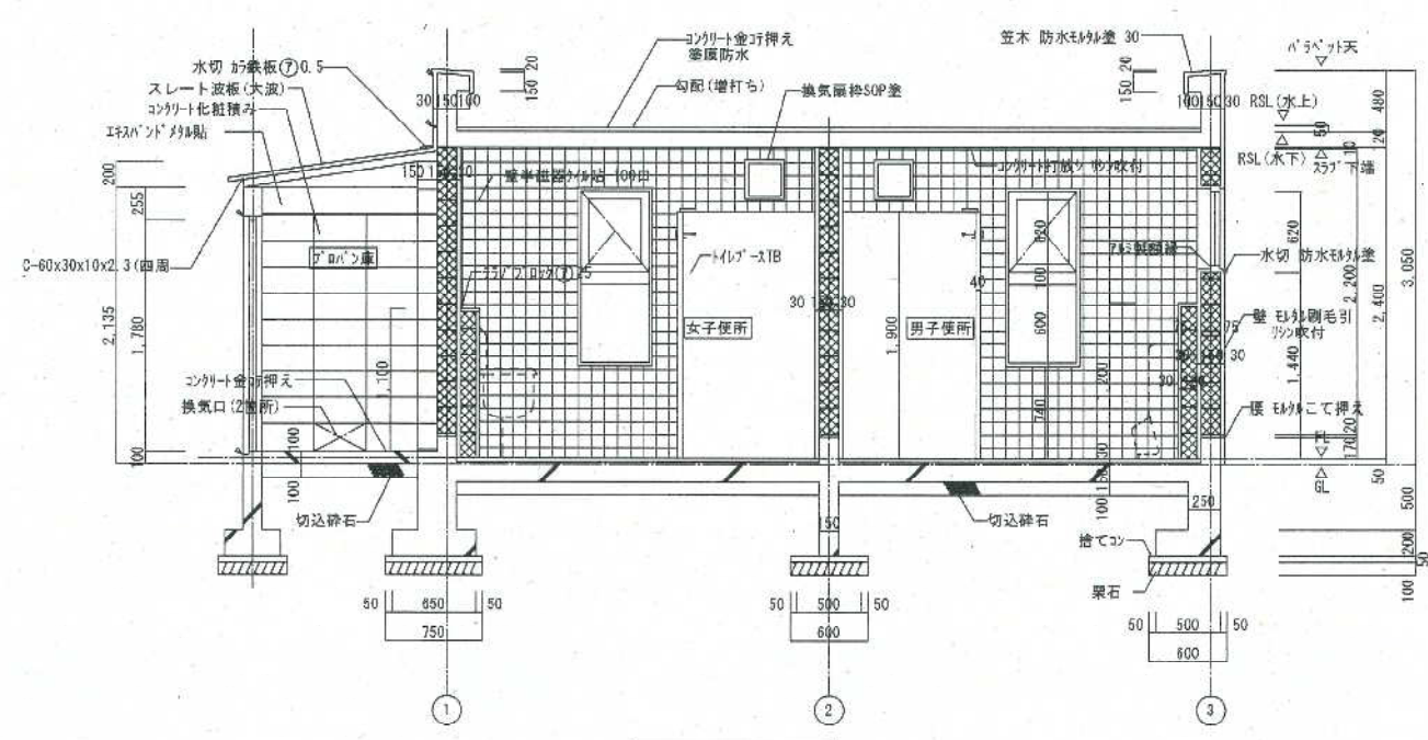
断面図 1:30
