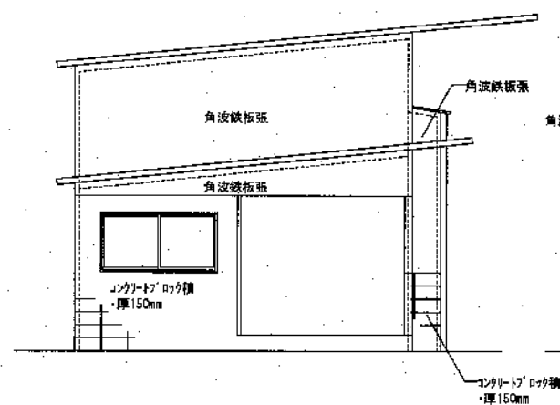
西立面図 1:50
