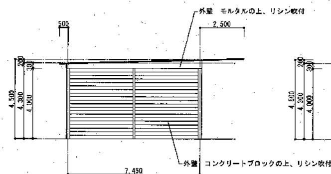
西立面図 1:100
