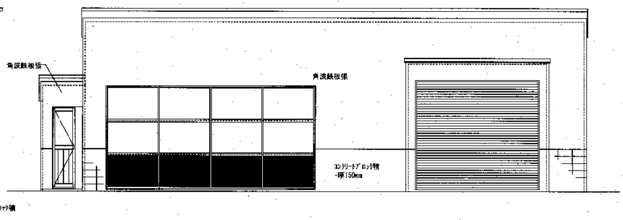
南立面図 1:50
