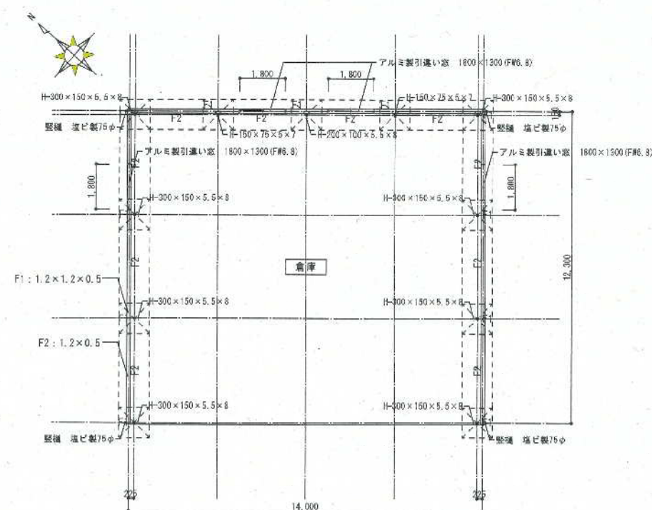
平面図 1:100
