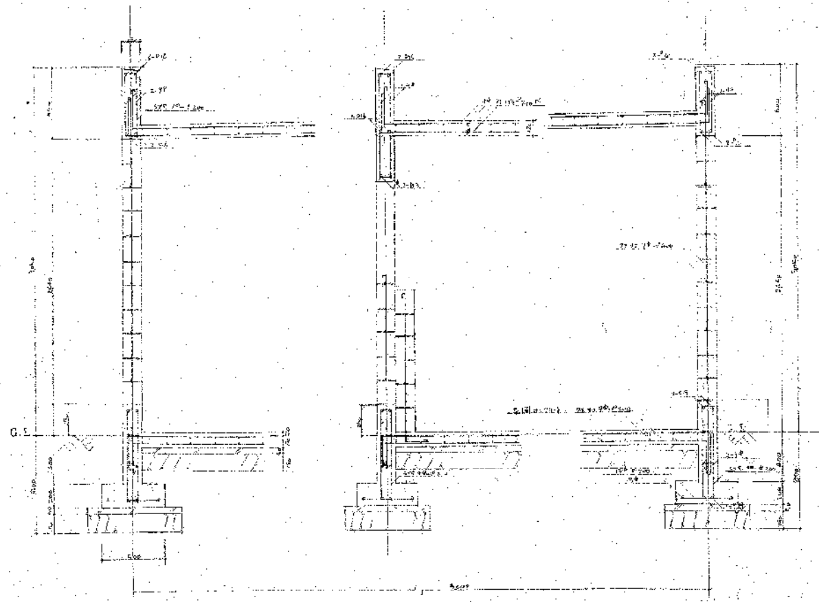
断面図 1:20
