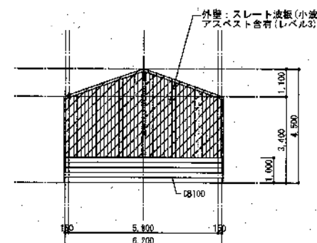
北立面図 1:100
