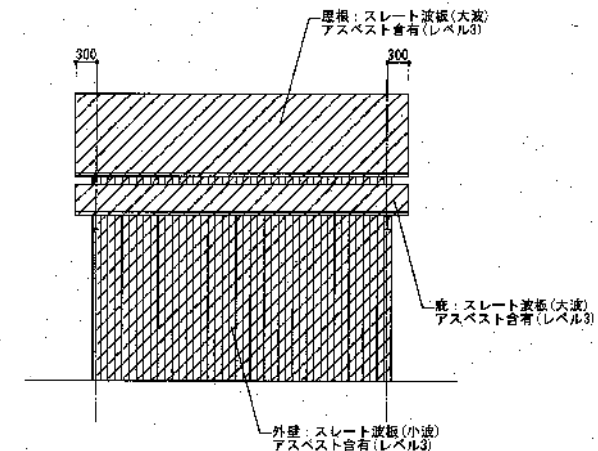
A棟 南立面図 1:50
