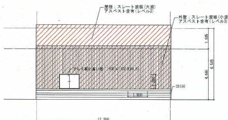
北立面図 1:100
