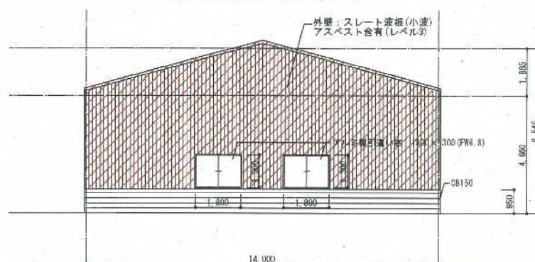
東立面図 1:100
