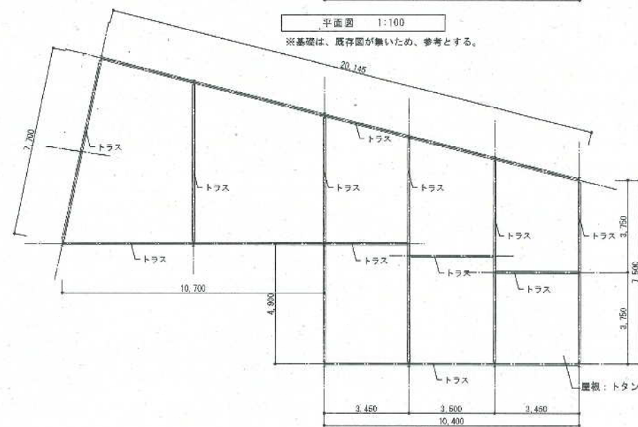
天井伏図 1:100
