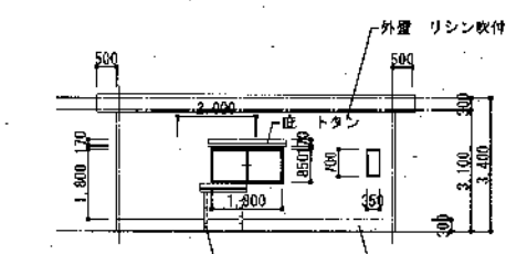
北立面図 1:100
