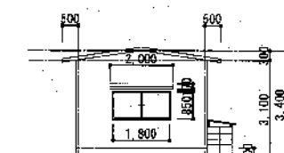
東立面図 1:100
