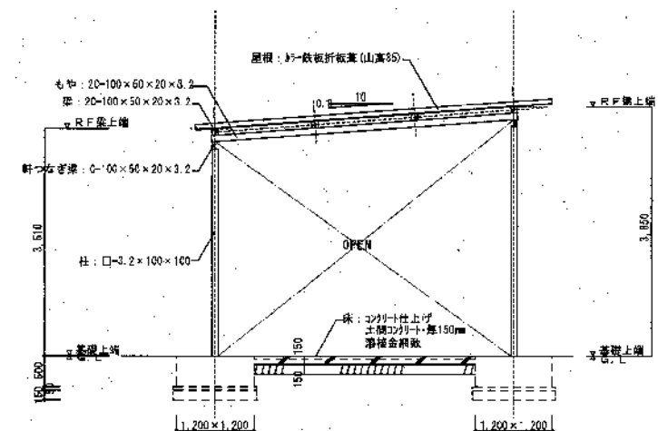
断面図 1:50
