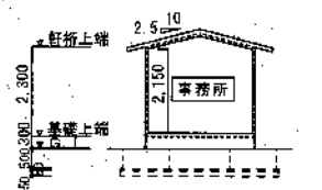
断面図 1:100
