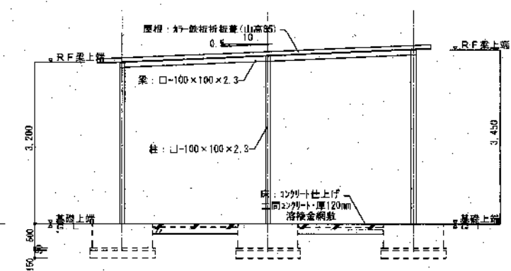
B棟 断面図 1:50
