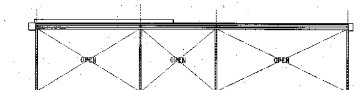
東立面図 1:100
