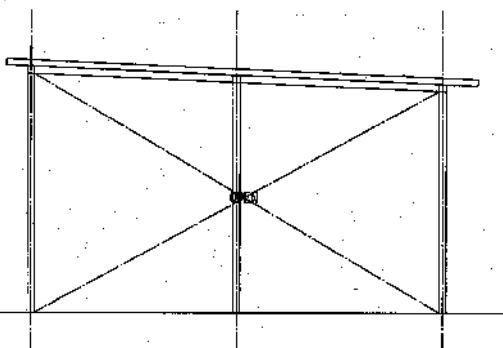
B棟 西立面図 1:50
