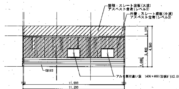
西立面図 1:100
