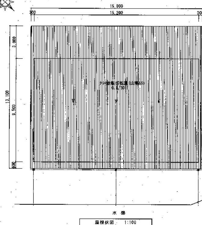
屋根伏図 1:100
