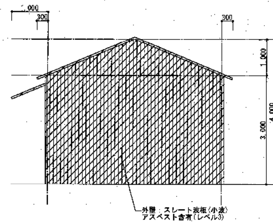
A棟 東立面図 1:50
