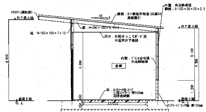
断面図 1:50
