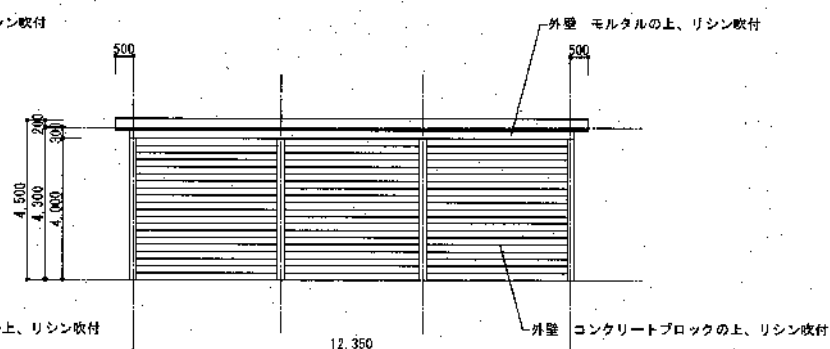
北立面図 1:100
