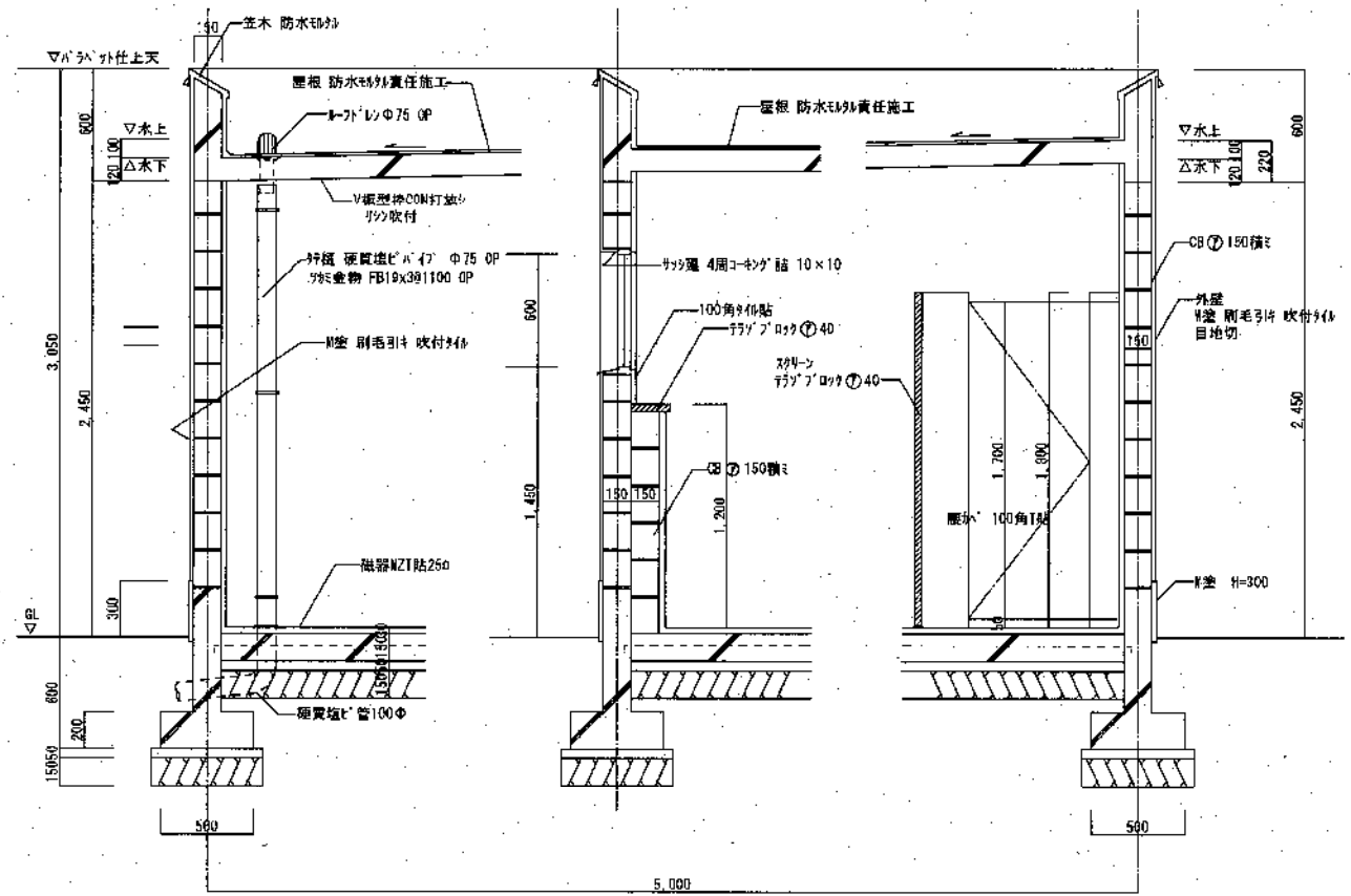
断面図 1:20
