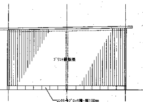
B棟 東立面図 1:50
