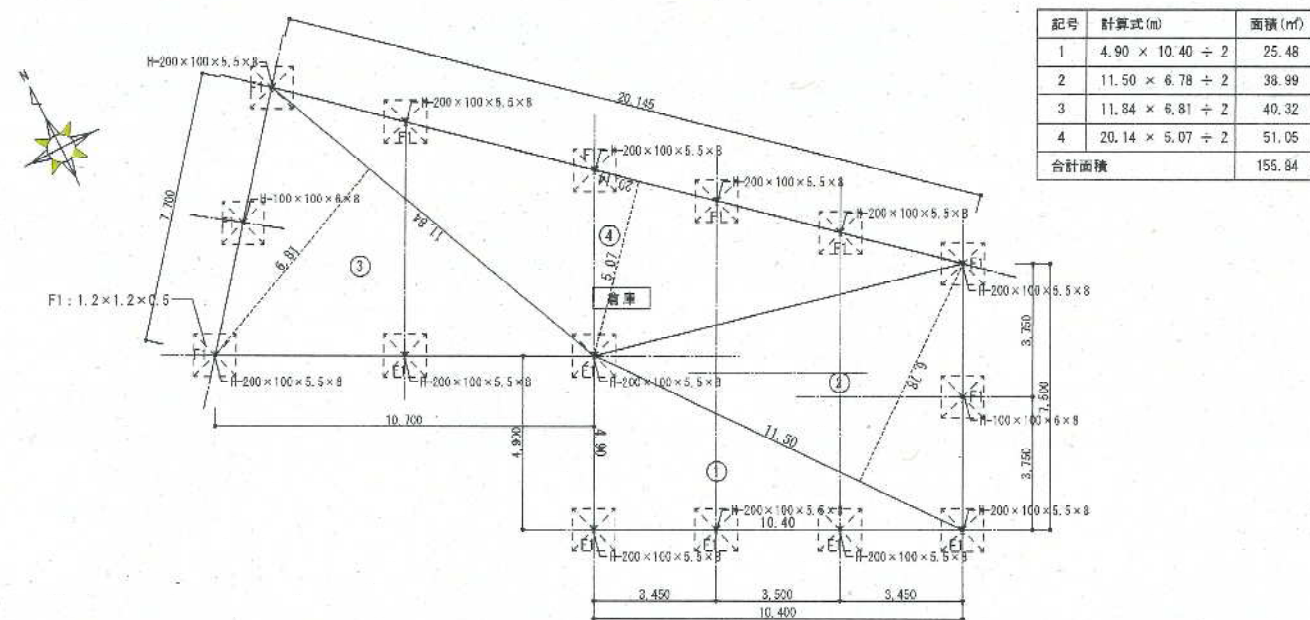
平面図 1:100 ※基礎は、既存図が無いので、参考とする。
