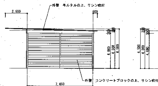
東立面図 1:100
