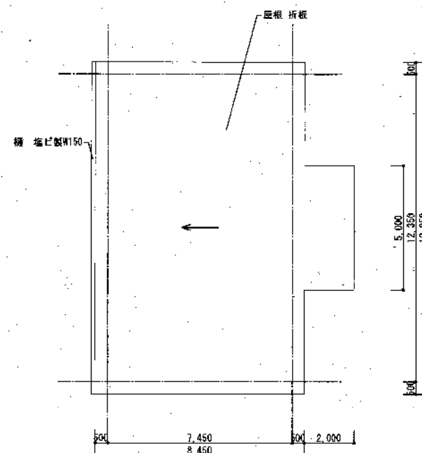
屋根伏図 1:100
