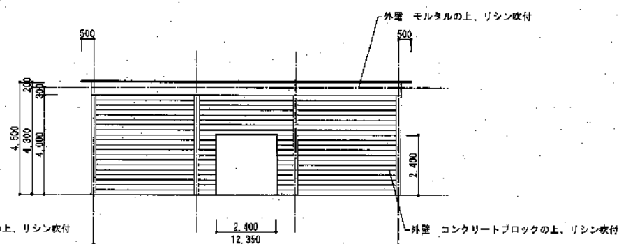
南立面図 1:100
