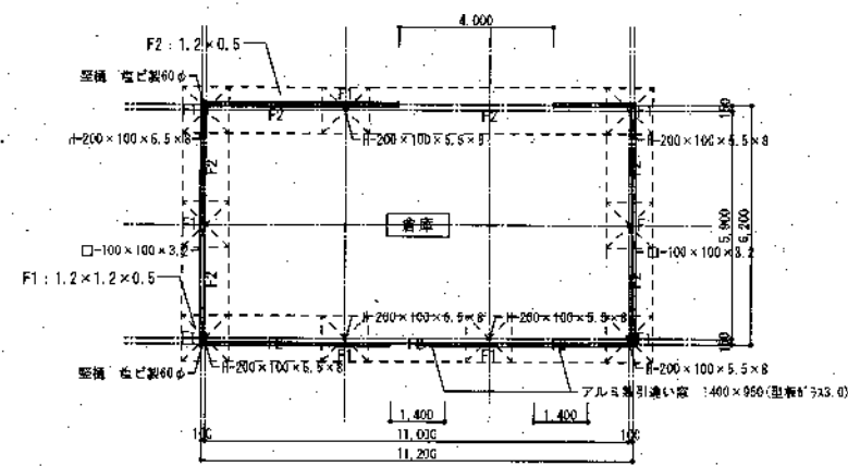
1階平面図 1:100
