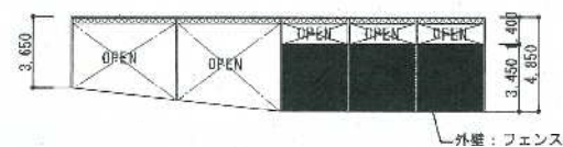
南立面図 1:200
