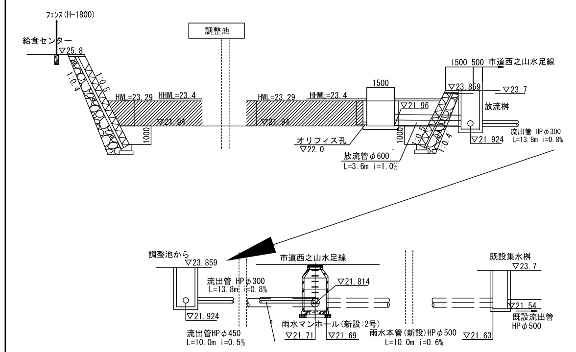
A断面図
