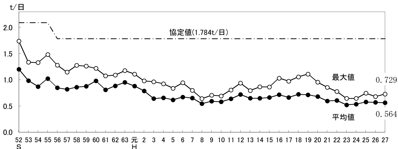
図-6 COD負荷量の推移
