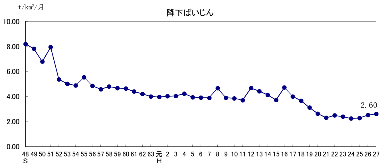
図－4 周辺地域（浜の宮、別府、播磨）における降下ばいじん総量の年間平均値
