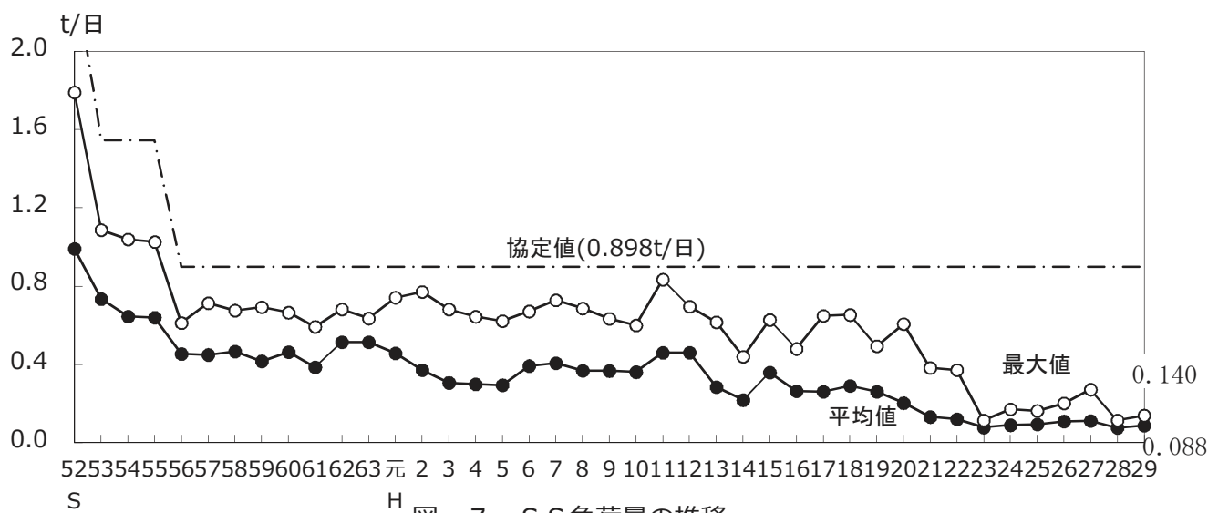
図-7 SS負荷量の推移
