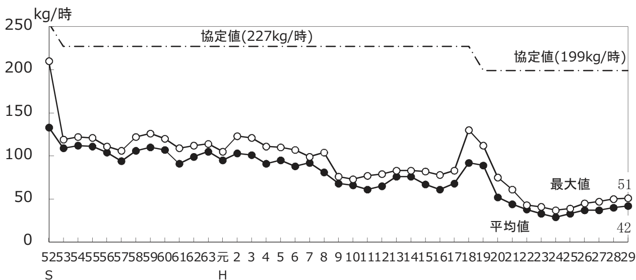
図－3 ばいじん時間排出量の推移
